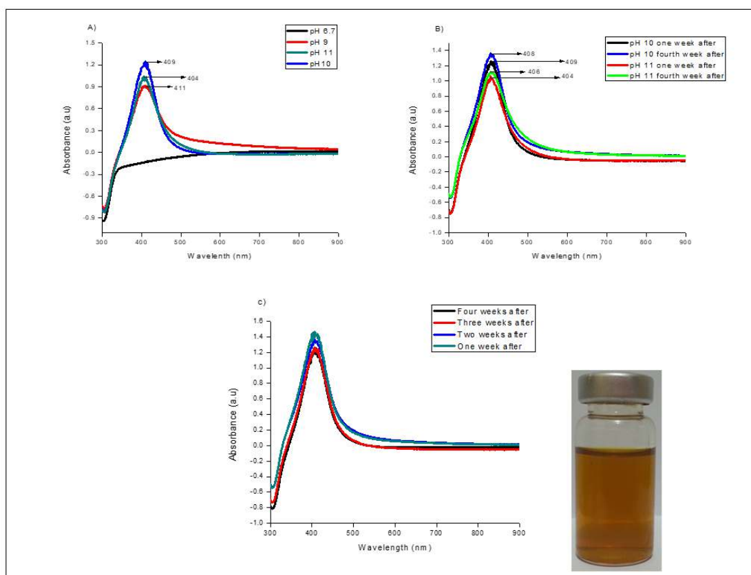
Figura 1. Formación de GC AgNps y espectrofotometría UV-visible
