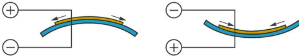
Fig 9. Transductor piezoeléctrico - Señal eléctrica (Mishra & Durgaprasad, 2016)
